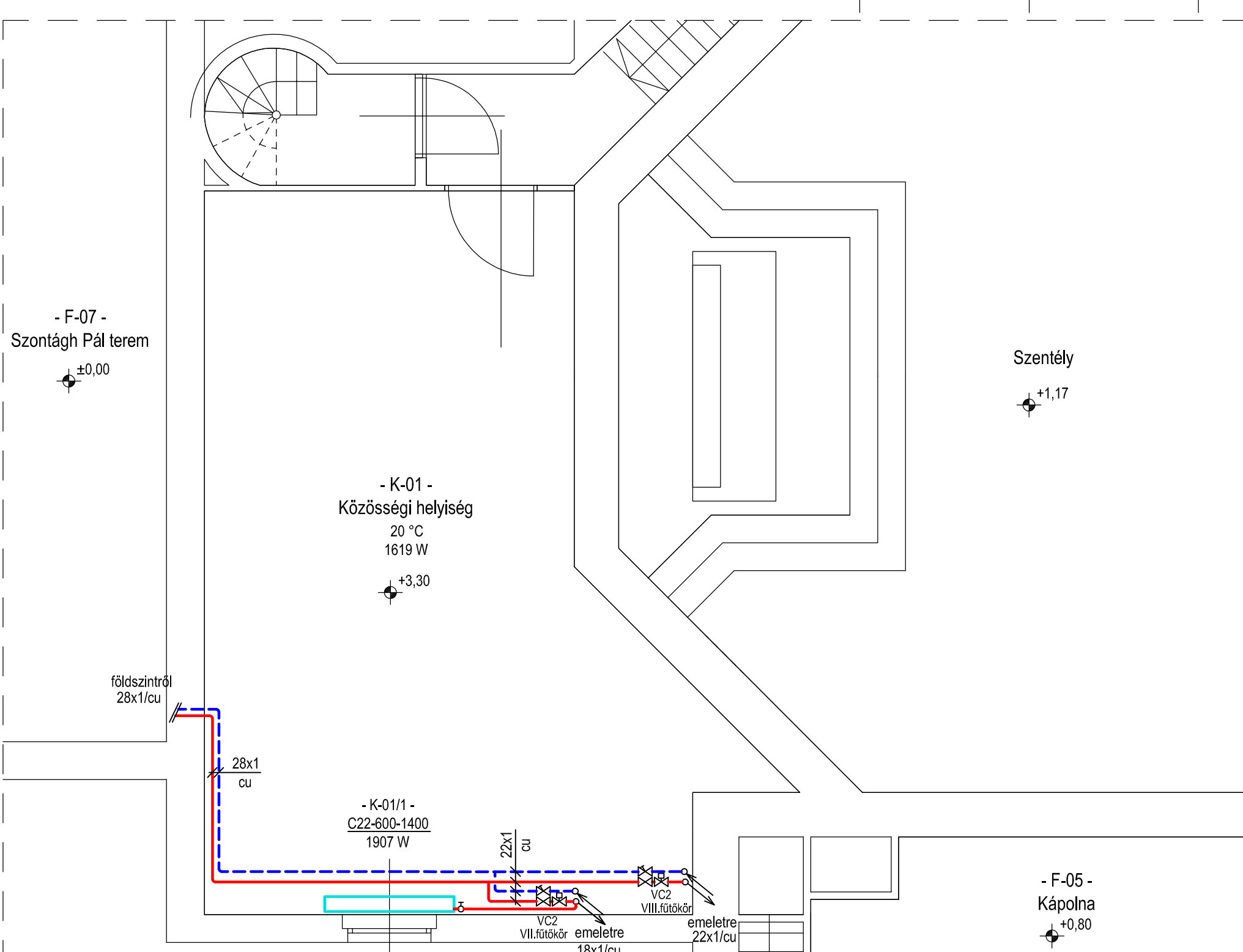
Félemelet alaprajz részlet M 1:50
